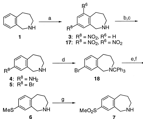
Scheme 1. Reagents and conditions: (a) KNO 3 , H 2 SO 4 ; (b) H 2 , PtO 2 , HCl; (c) NaNO 2 , HBr, CuBr; (d) PH 3 CCl, Et 3 N, DMAP; (e) n -BuLi, THF, −78 °C; (f) CH 3 SSCH 3 , 3 N HCl, Acetone; (g) CF 3 CO 3 H (2 equiv), CF 3 CO 2 H.
